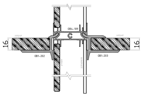
7 - DETAY
