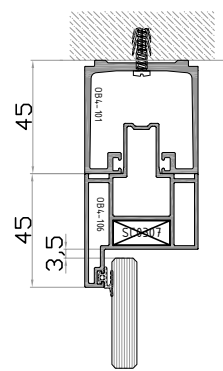
9 - DETAY
