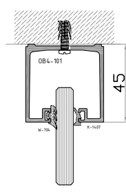
10 - DETAY
