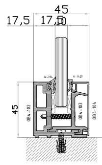
8 - DETAY
