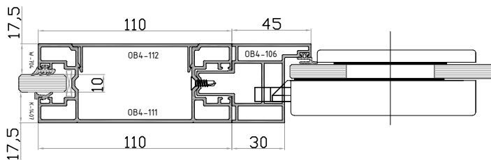
3-DETAY
