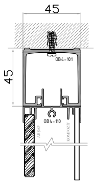
6 - DETAY
