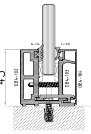
11 - DETAY
