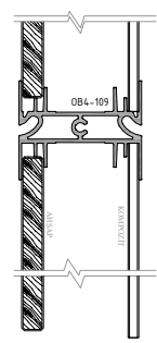
7 - DETAY
